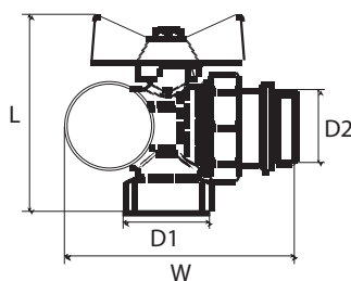
Zawór z śrubunkiem Brass KHT 1" kątowy z uszczelką + termometr (niebieski, czerwony)
