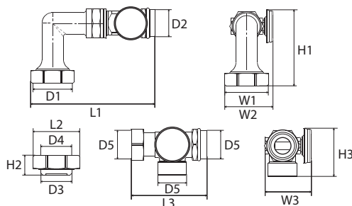
Grupa pompowa Brass KHT nieuzbrojona / GP-B-B
